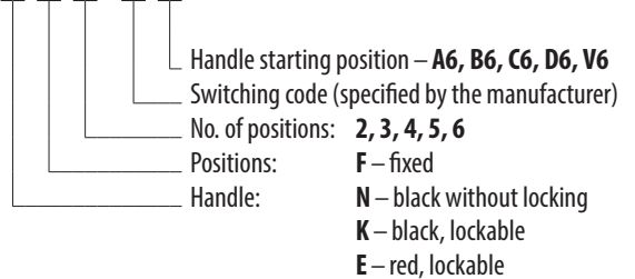
XSV10-A F . . . . .
