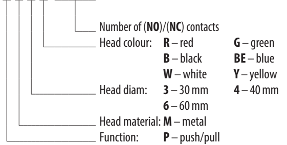
XMB10-A . . . . .NO/.NC
