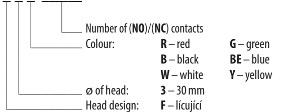
XPB10-A F 3 . . .NO/.NC
