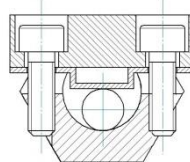
Upevnění kabelu o průměru do 10mm
