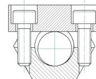
Upevnění kabelu o průměru nad 10mm
